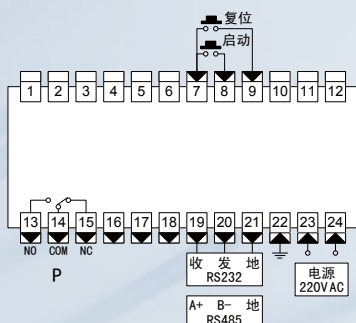
■ A规格160×80尺寸仪表
