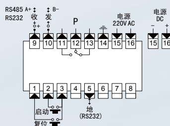
■ D规格96×48尺寸仪表
